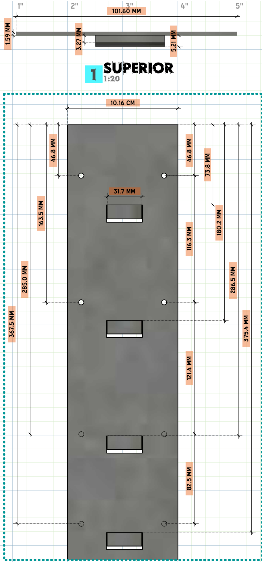
18 DETALLE B
